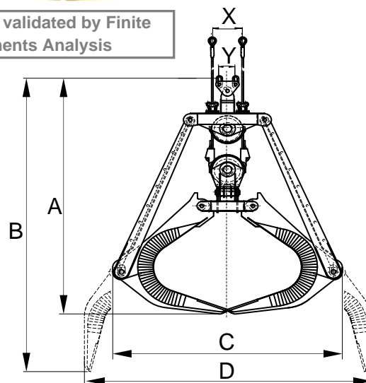
PNA-1,8
